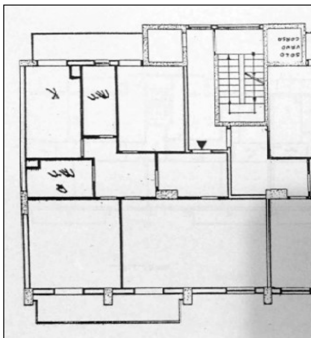
Stralcio della planimetria del piano tipo dell'edificio 6/2, scala A, allegata all'istanza di N.O. provvisorio di prevenzione incendi pratica n. 46707 del 20.12.1990
