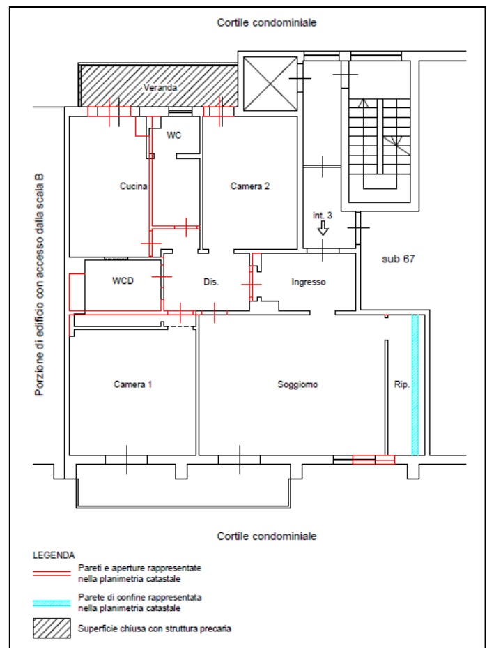
Planimetria catastale dell'immobile e planimetria dello stato di fatto con l'indicazione delle difformità rispetto alla planimetria catastale
